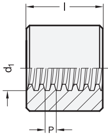
单线螺纹
